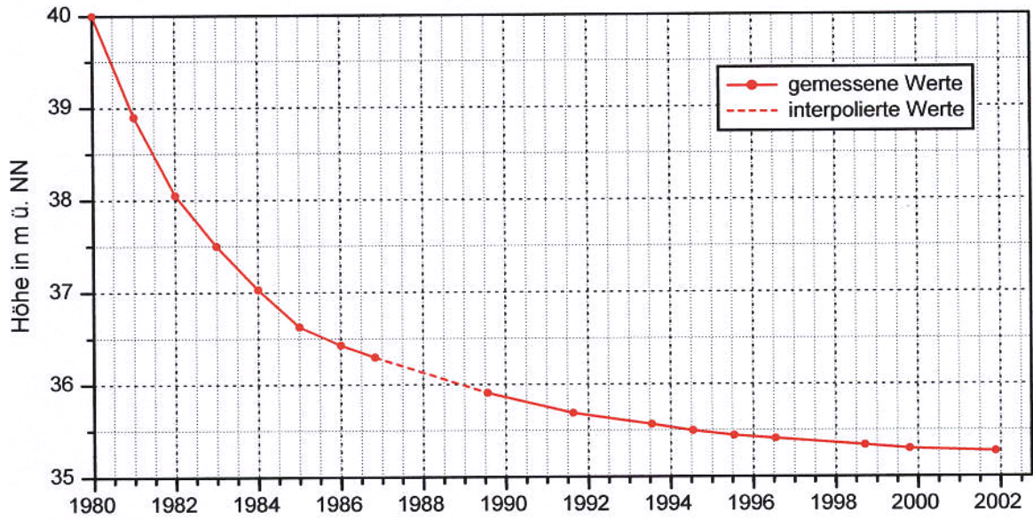
Abbildung 3: Setzungen des Kuppenbereiches der Deponie Georgswerder
