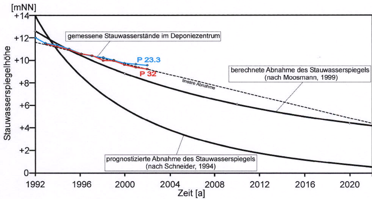
Abbildung 6: Prognostizierte und gemessene Abnahme des Stauwasserspiegel im Deponekörper (Quelle: Moosmann GLA Hamburg)
